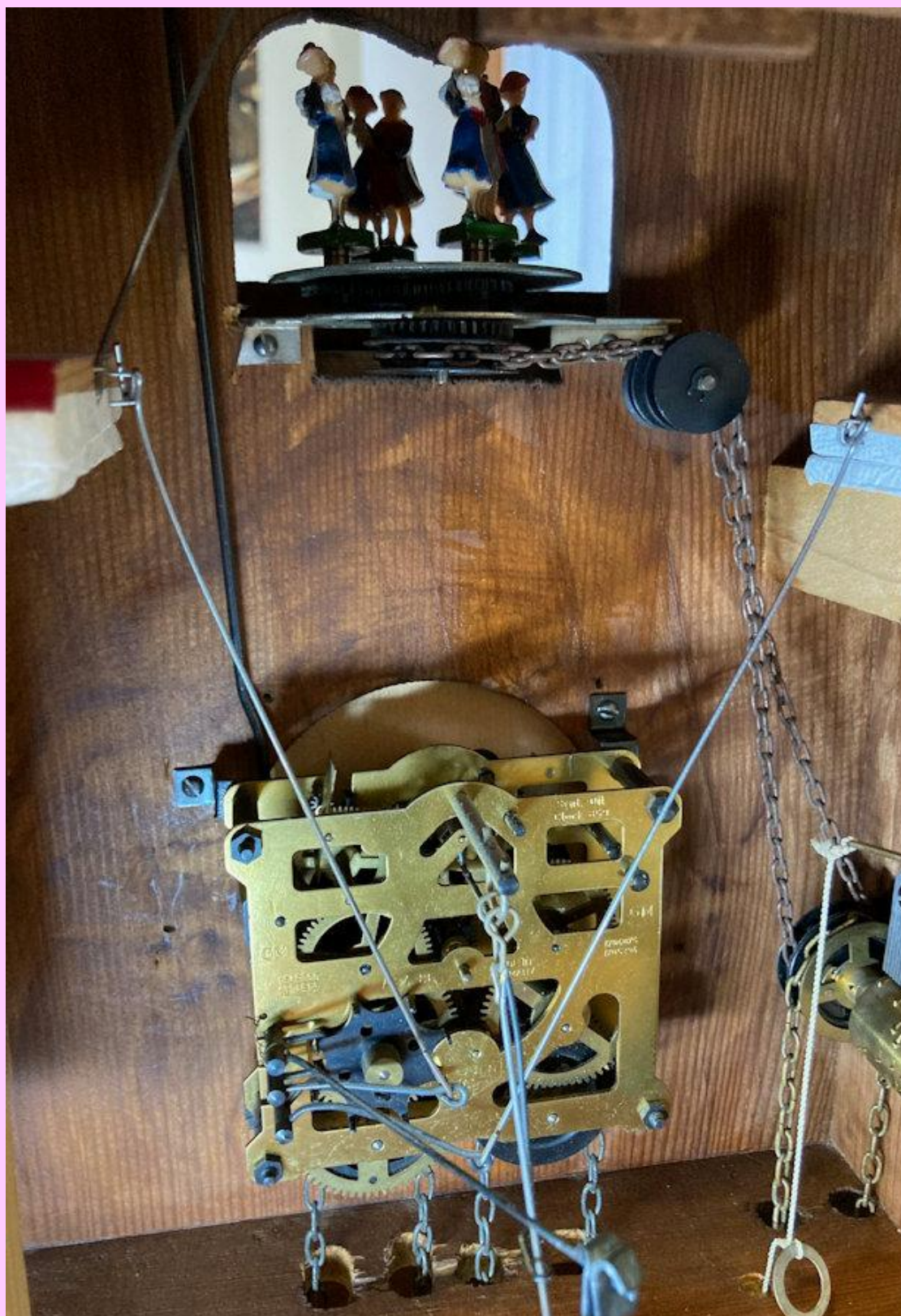
Il retro del cucù con parte del carillon ed il cordoncino per farlo funzionare indipendentemente dal meccanismo
