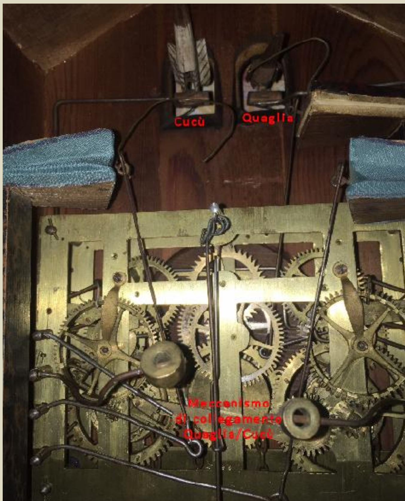
L'interno del cucù
