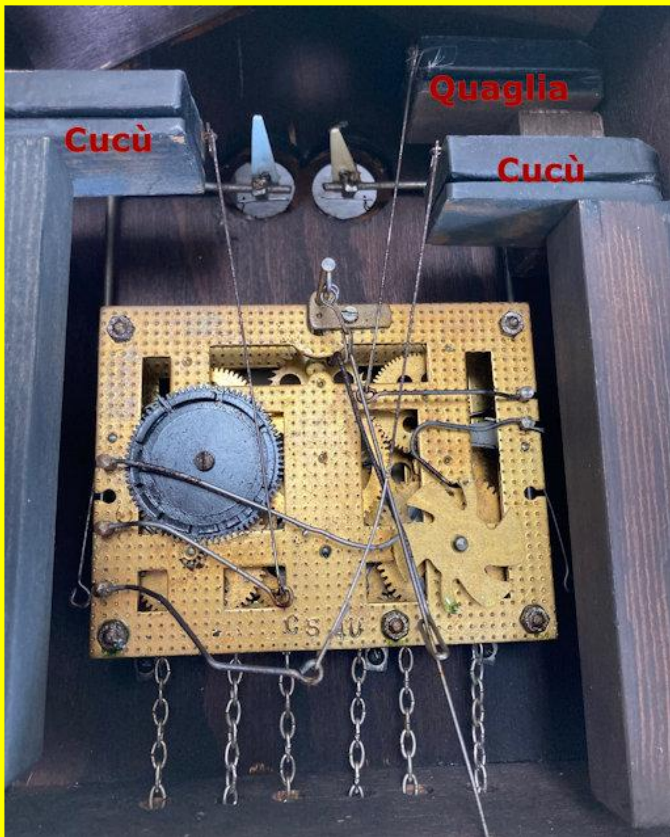
Il meccanismo con in evidenza i due mantici per il cucù e quello per la quaglia
