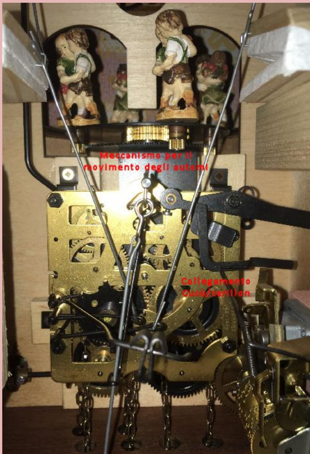
L'interno del cucù
