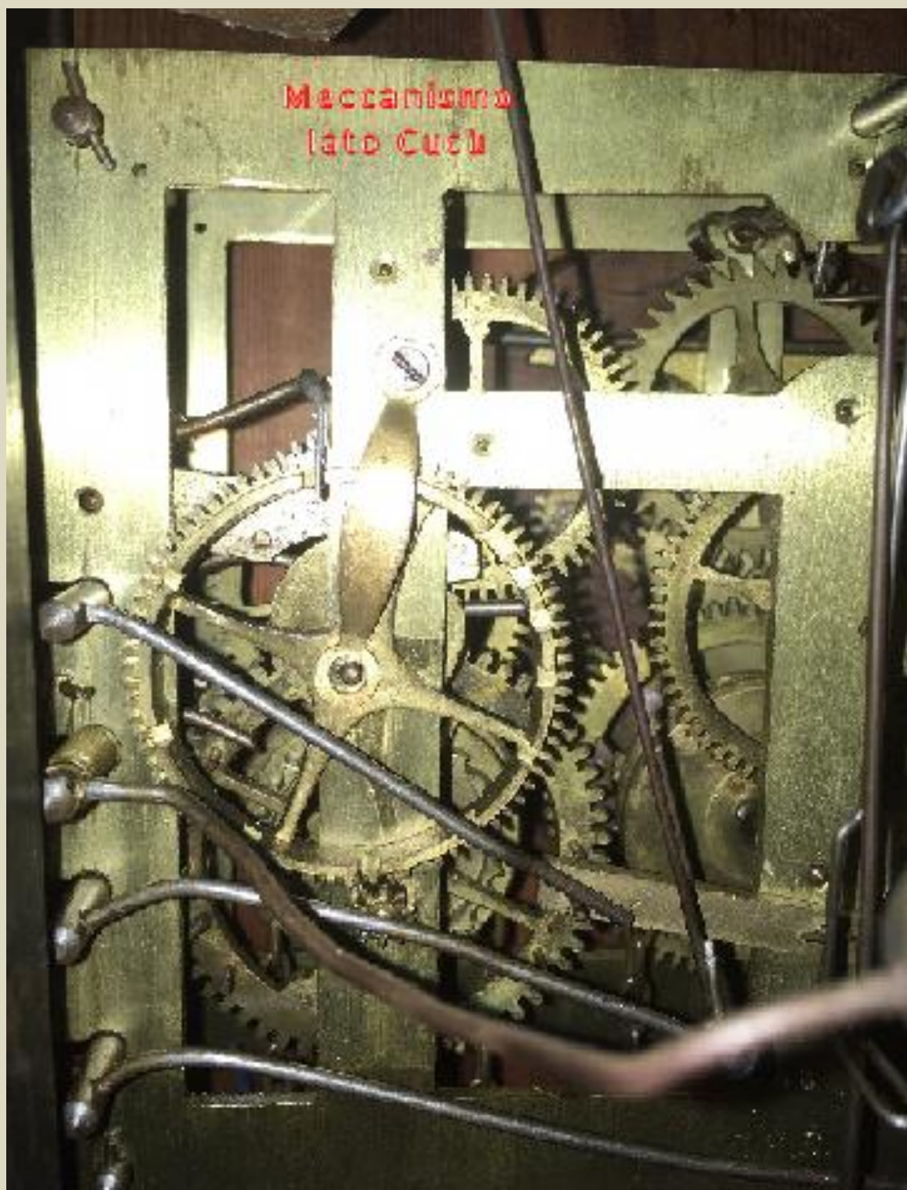
Particolare meccanismo del cucù
