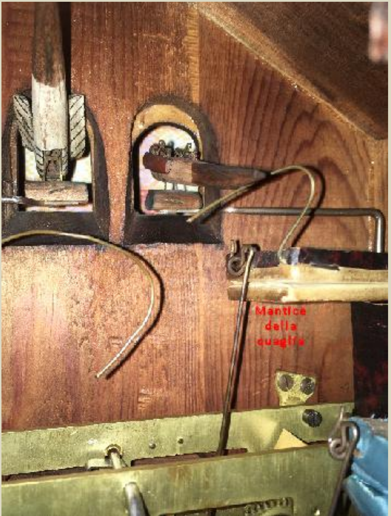
Parte alta dell'interno del cucù
