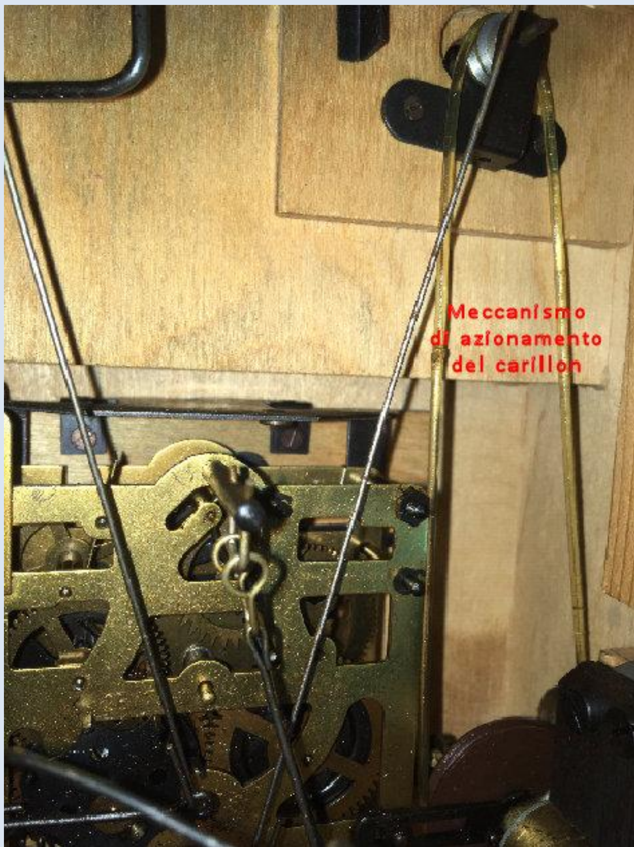
Particolare dell'interno del cucù
