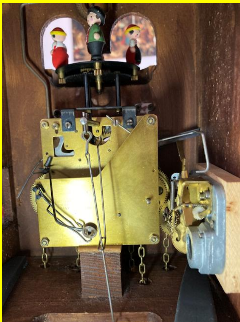
Il retro del cucù con il carillon. Si nota un sostegno del meccanismo all'interno del quale passa una delle catene del carillon.
